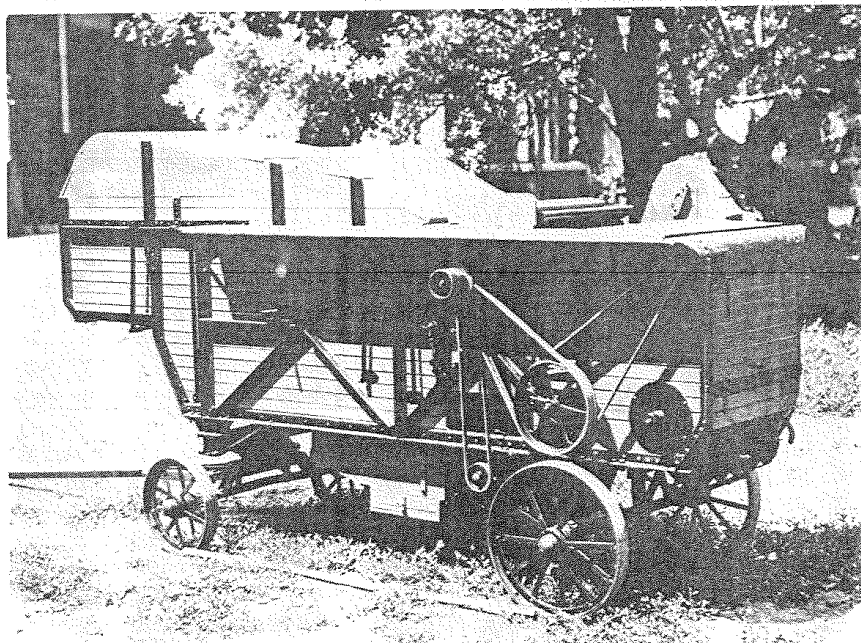
8-as, acélvázás cseplőgép 1930 körül (modell)
